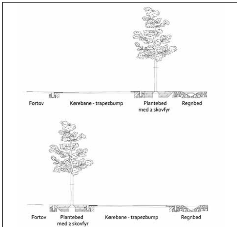
Tværsnit af vejen.
