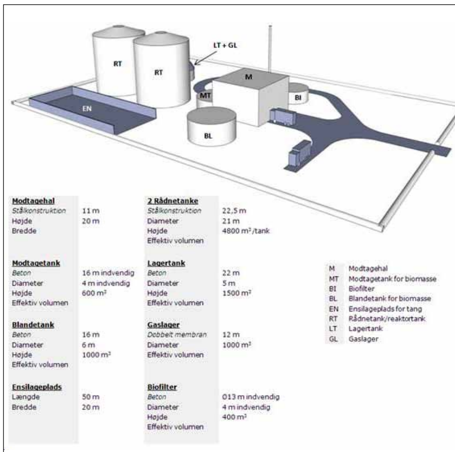
Anlægsdesign med betegnelser.
